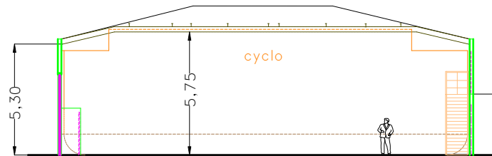
Coupe AA
