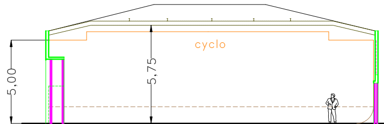
Coupe AA
