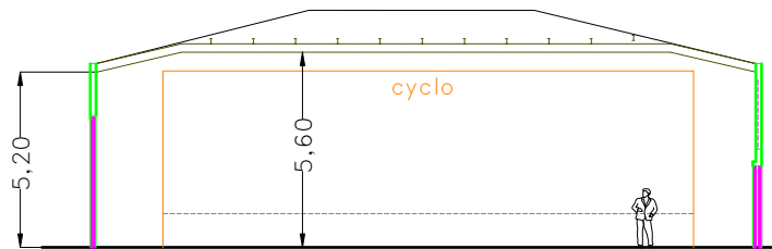
Coupe AA
